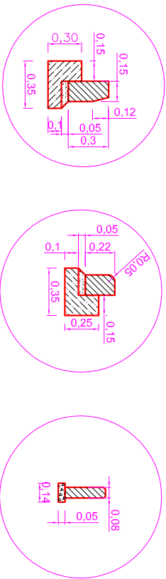
PRZEKROJE SZCZEGÓŁOWE KRAWĘŻNIKÓW I ŁAW
